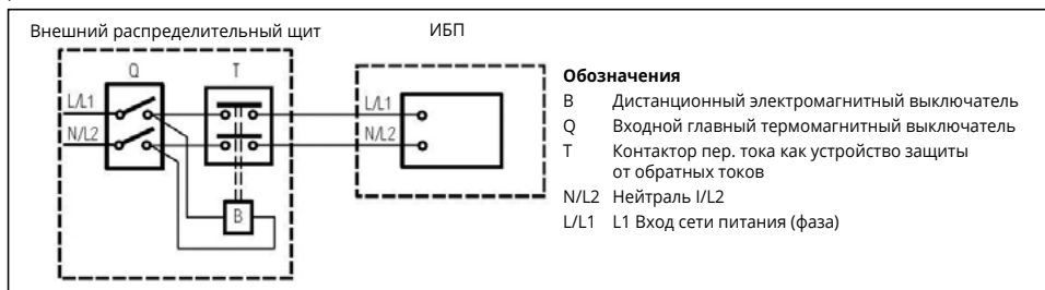
Проводка внешней системы защиты от обратного питания
